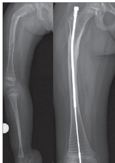
Figura 2. Antes y después del enclavamiento intramedular.
